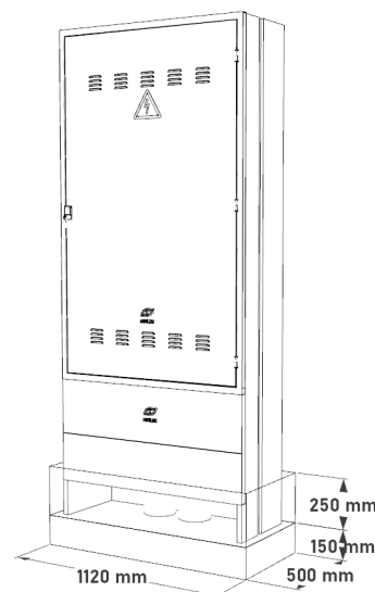
Excavación en función del modelo
